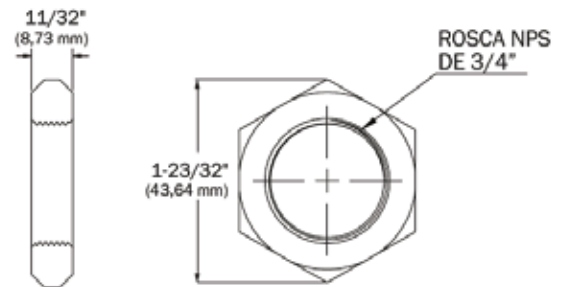
Tuerca de fijación
