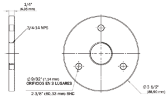
Brida de montaje de fijación (perno a recipiente).
