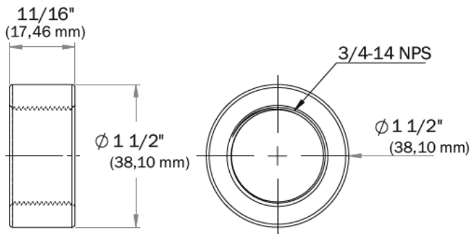
Acoplamiento de montaje (soldadura a recipiente).
